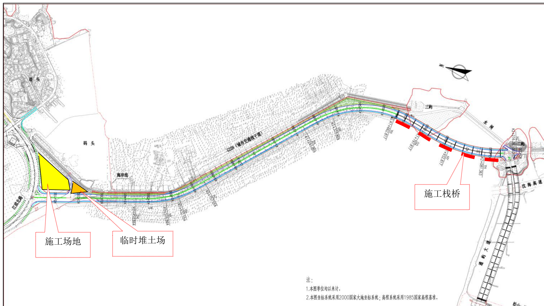
图2.10-1 本项目临时工程布置示意图
