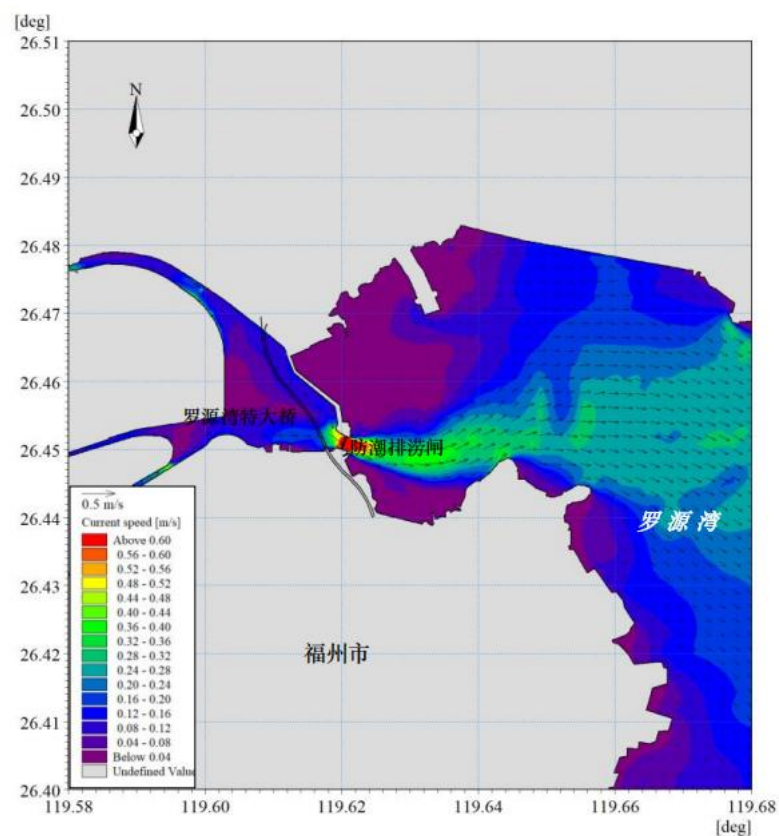
图4.1-15 工程附近海域现状潮流场（闸门开启，落急时）
