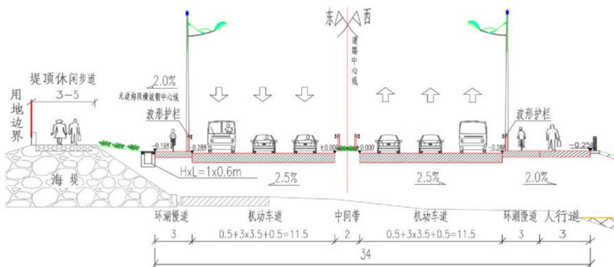
图 2.5-1 标准路段路基横断面图
