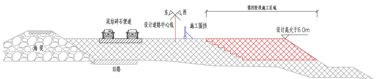
第四阶段填筑示意图
