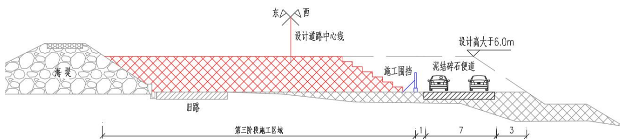
第三阶段填筑示意图
