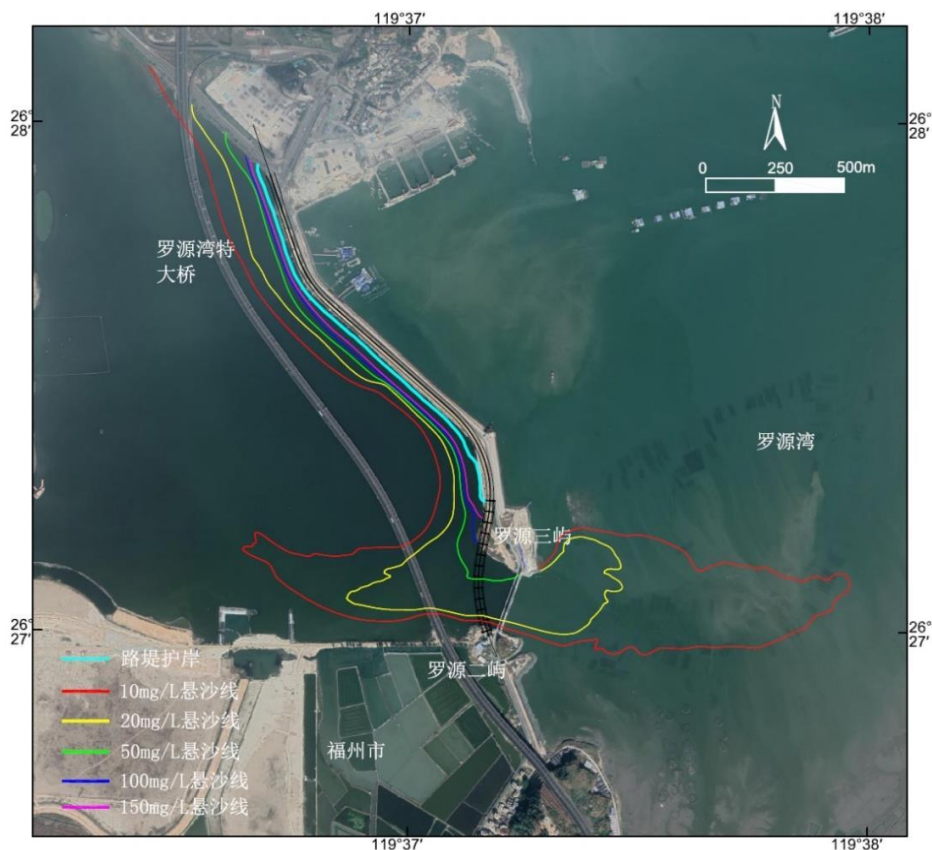
图4.1-49 护岸施工作业悬浮泥沙最大扩散范围图（闸门开启）
