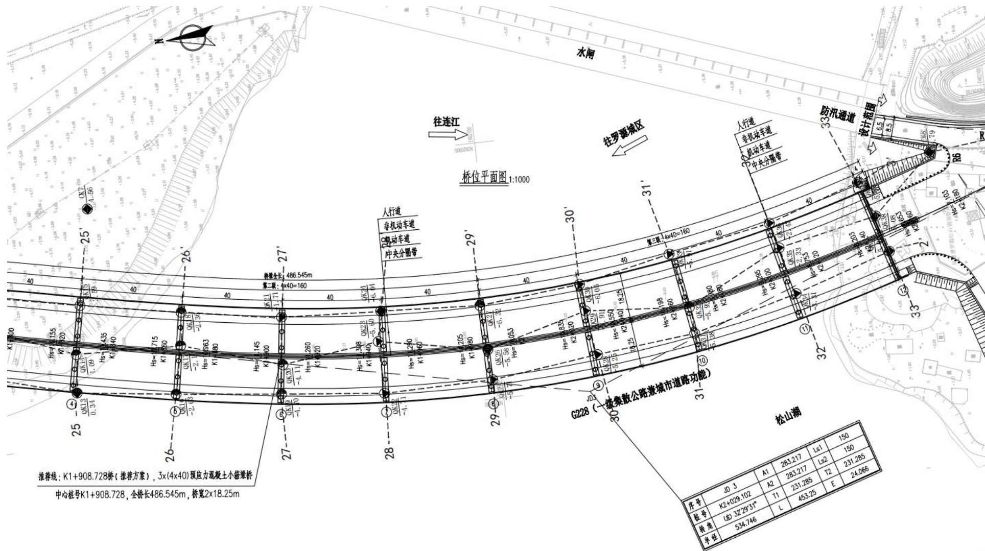
图 2.5-11 2 号桥桥位平面图 (2)
