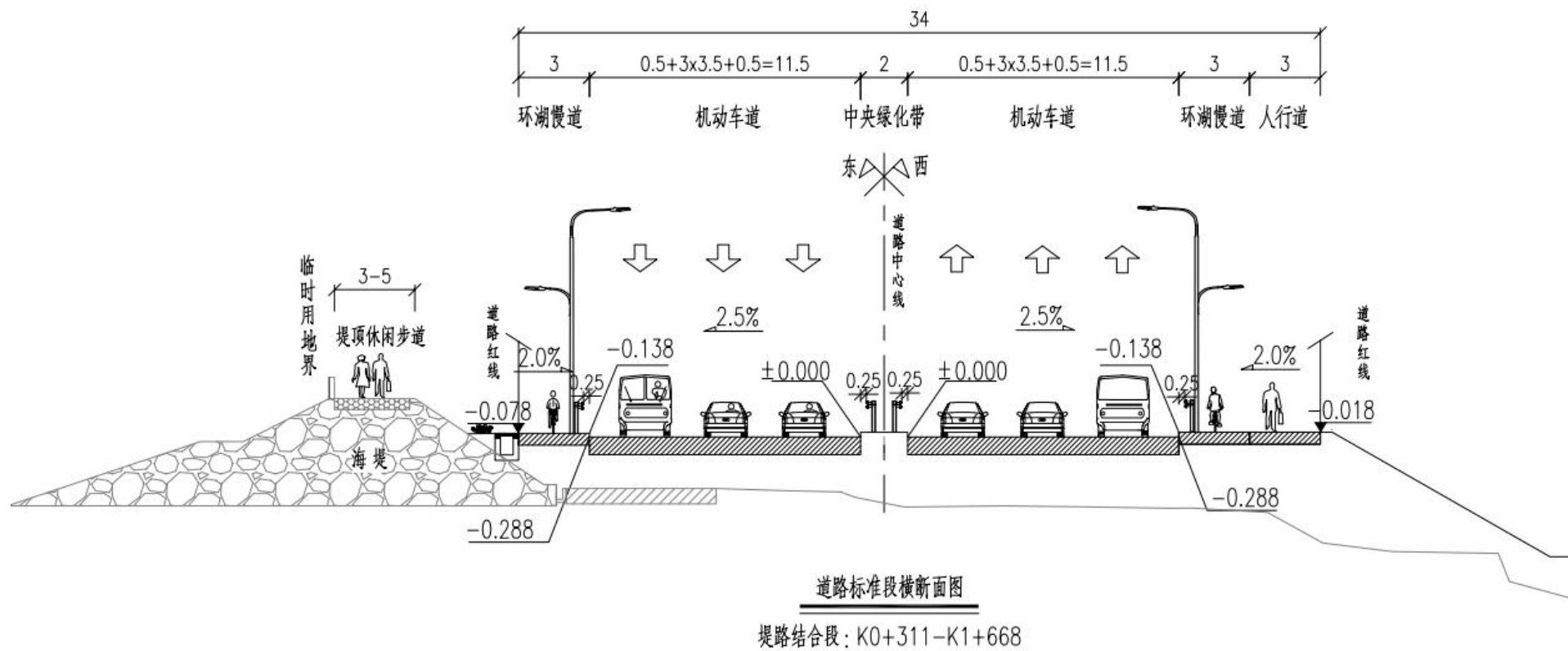
图 2.5-5 K0+311~K1+668 段路基标准横断面图
