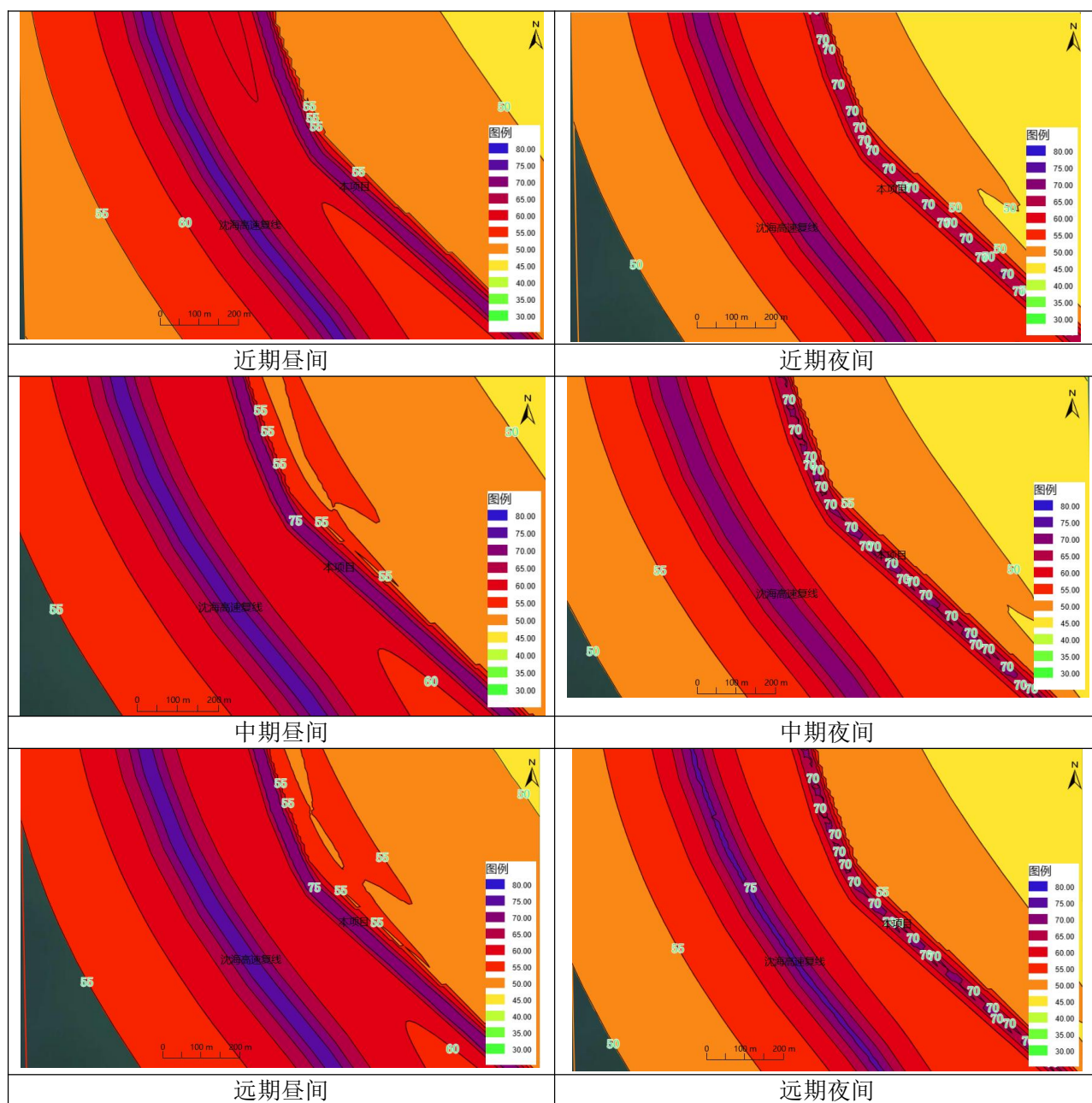
图4.2-8 营运期水平向交通噪声等声值线图（叠加高速公路交通噪声影响）
