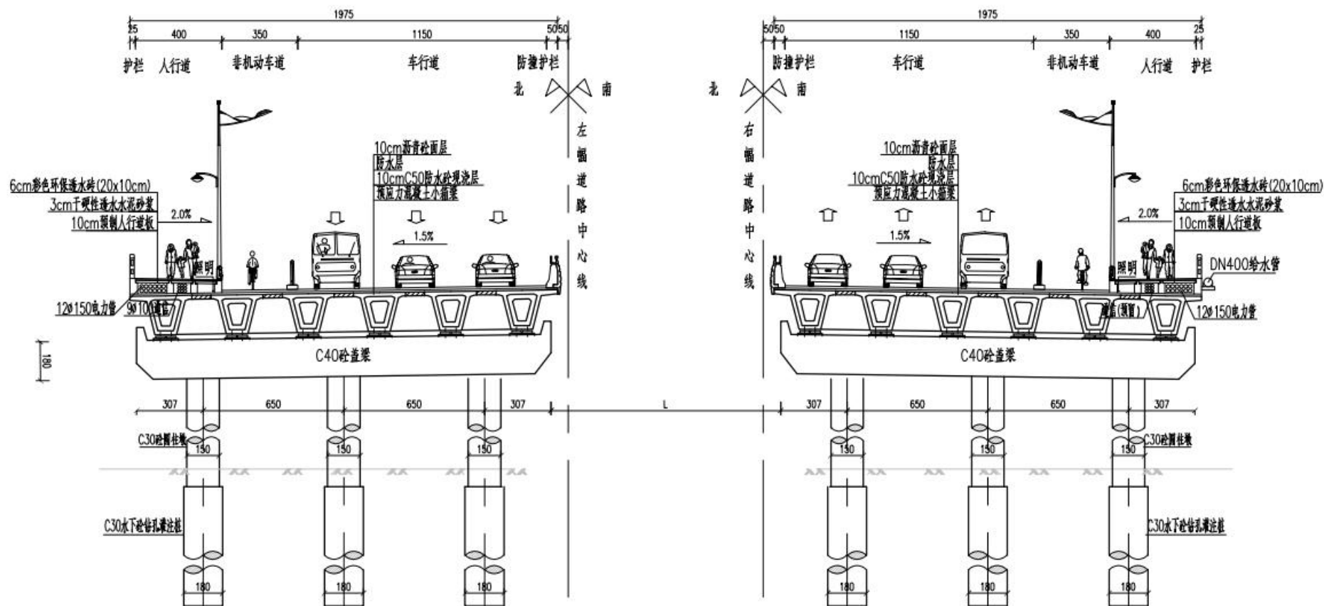
桥墩处横断面图 (跨高速处)
