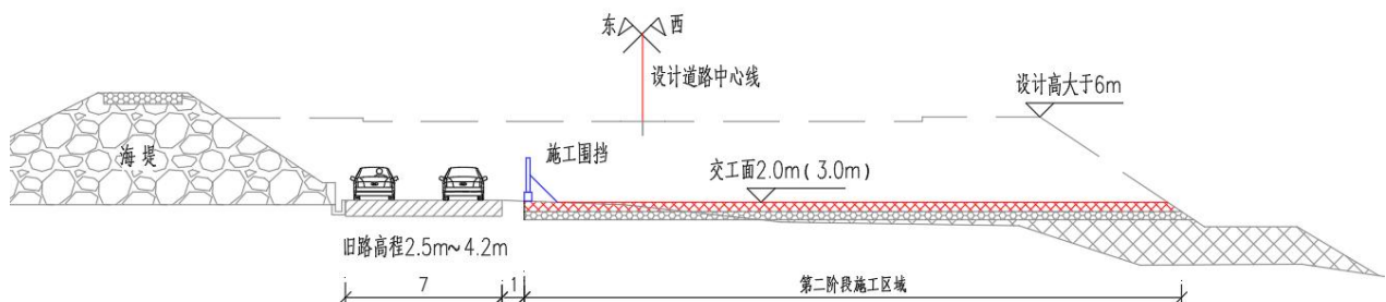
第二阶段填筑示意图
