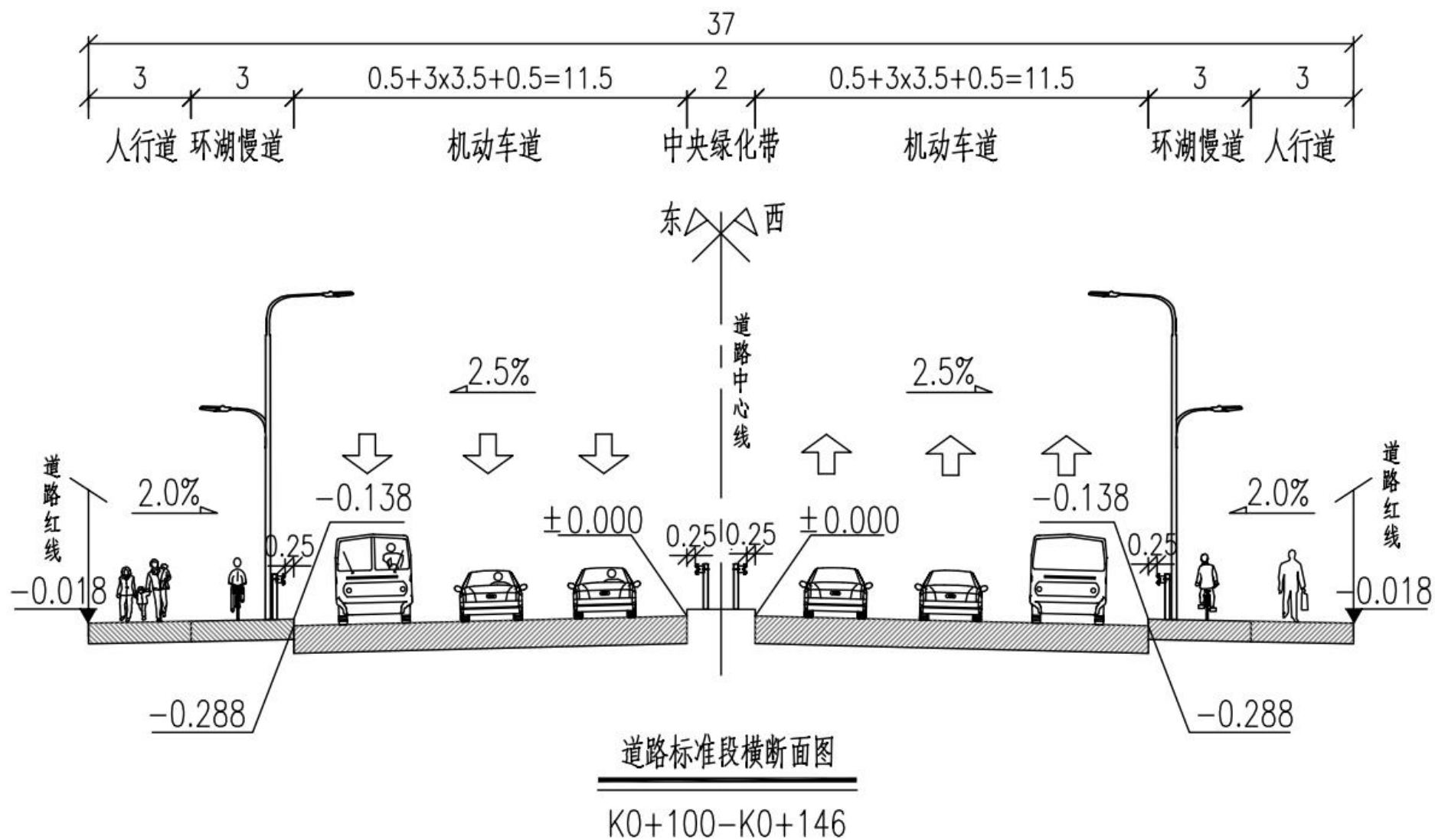
图 2.5-2 K0+000~K0+146 段路基标准横断面图
