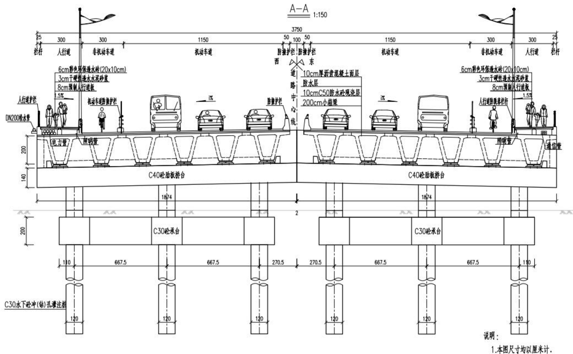
图 2.5-12 2号桥桥型布置图
