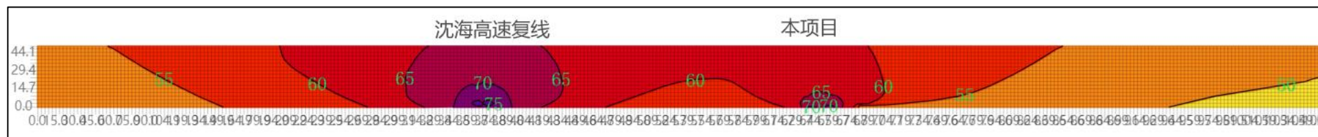
图 4.2-11 营运中期交通噪声铅垂向分布图
