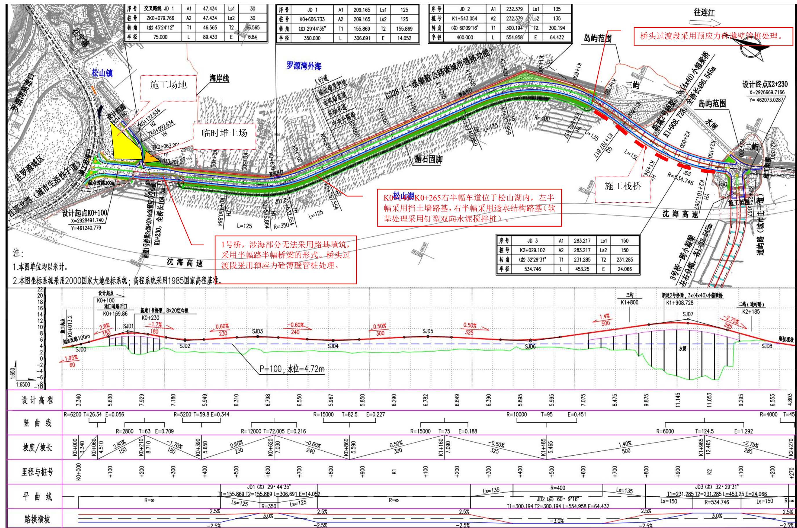
图 2.2-6 本项目总平面布置图
