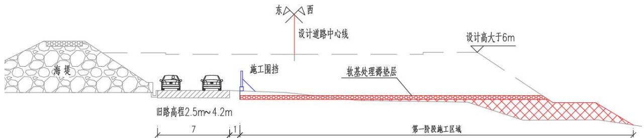
第一阶段填筑示意图
