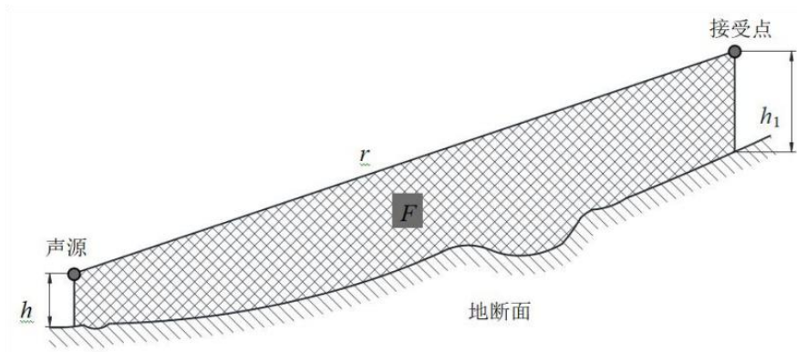
图4.2-4 估计平均高度 h_m 的方法
