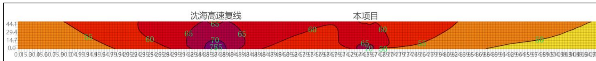
图 4.2-10 营运近期交通噪声铅垂向分布图
