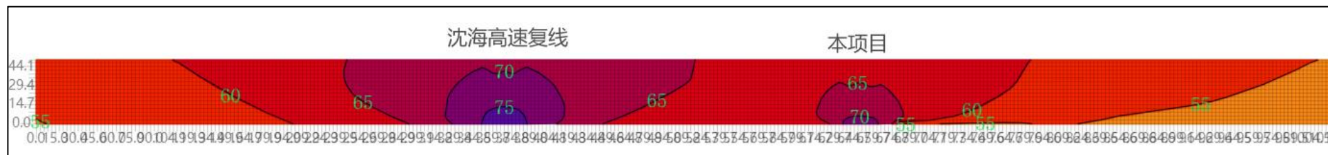
图 4.2-10 营运近期交通噪声铅垂向分布图
