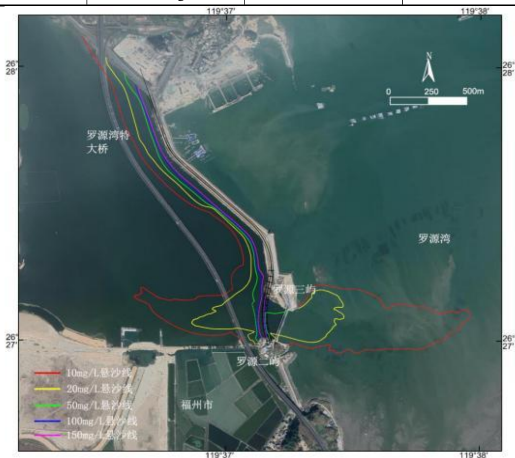
图4.1-52 整个项目产生的悬浮泥沙影响最大范围包络图（闸门开启）
