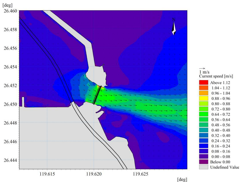
图4.1-20 工程附近海域现状潮流场（低水位落潮时开闸泄洪，60分钟后）
