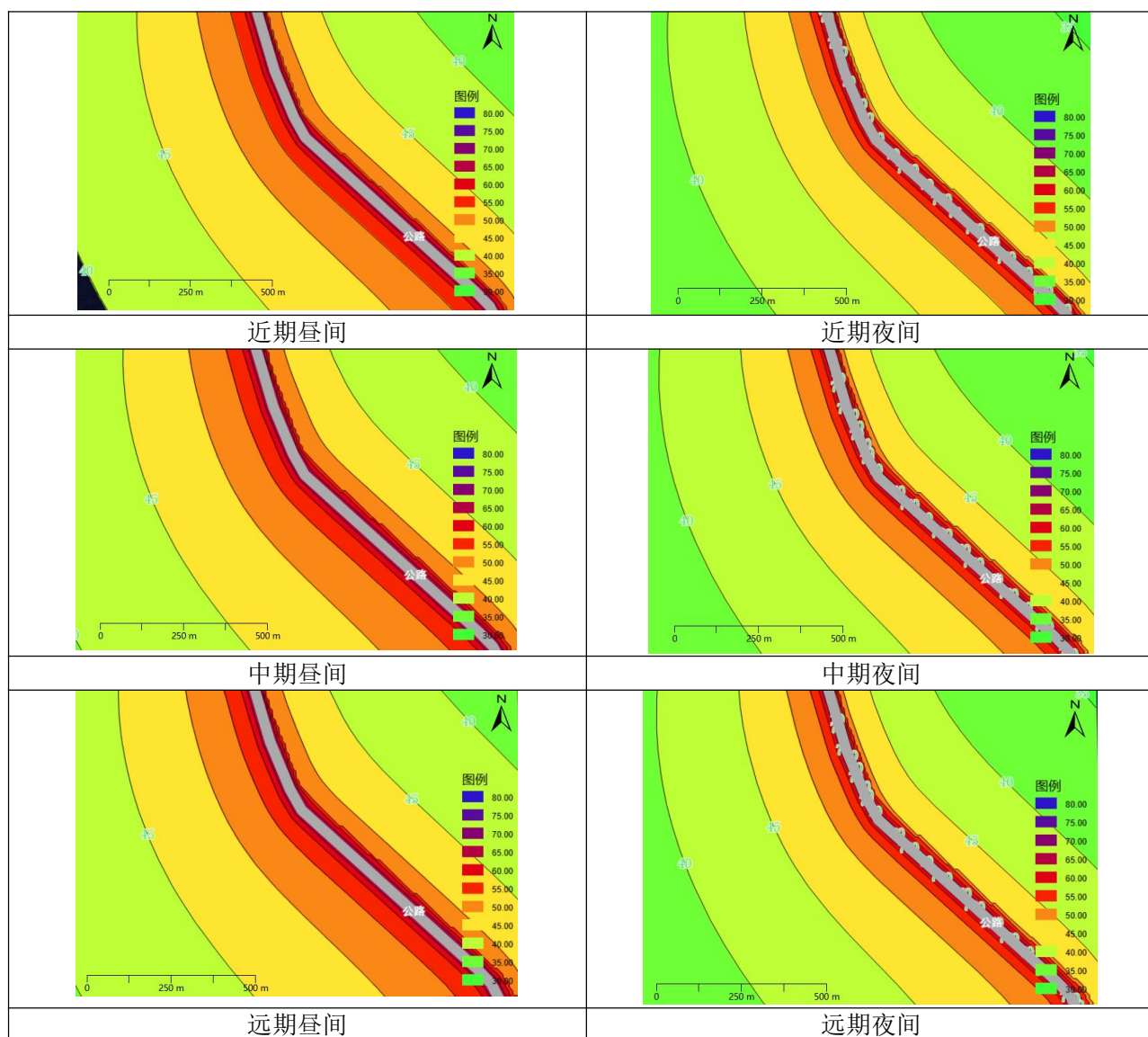
图4.2-7 营运期水平向交通噪声等声值线图（未叠加高速公路交通噪声影响）
