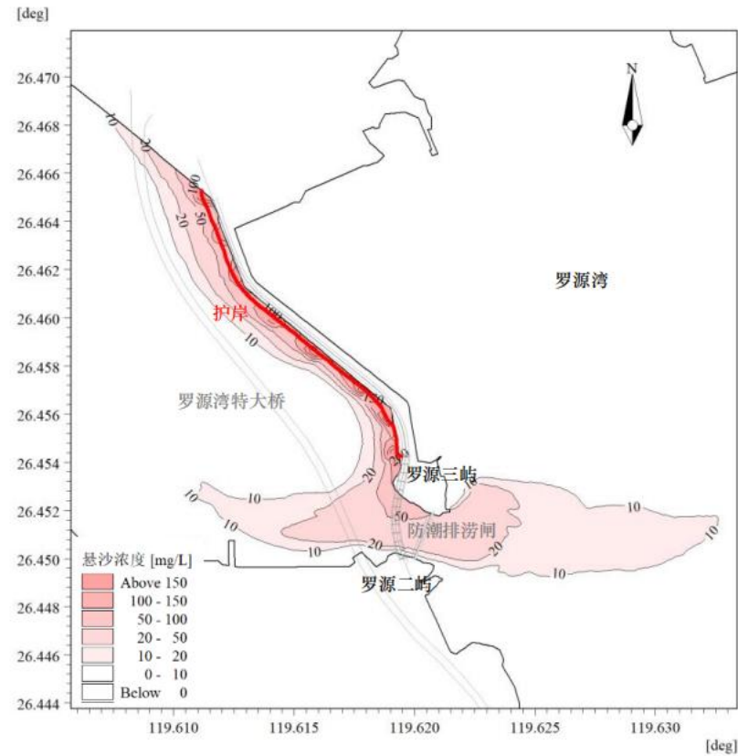
图4.1-48 护岸施工悬浮泥沙各预测点扩散范围图（闸门开启）
